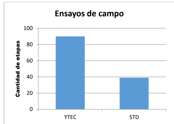
Fig. 2: Durabilidad de pistones ensayados
