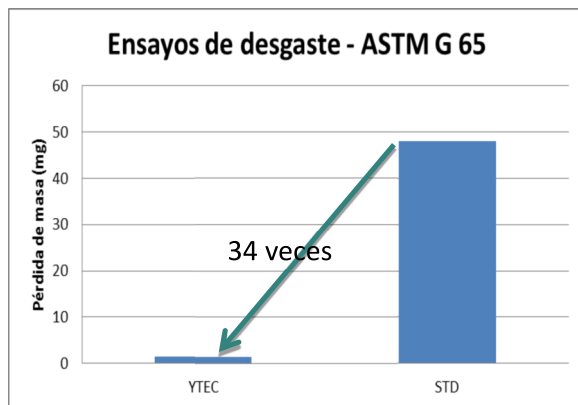
Fig. 1: Pérdida de masa en ambos materiales
